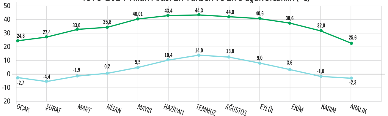
1975-2024 Yılları Arası En Yüksek ve En Düşük Sıcaklık (°C)
